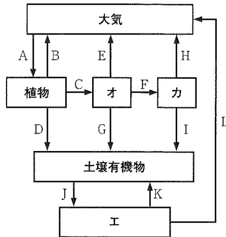
図1 陸上生態系における炭素循環の模式図
