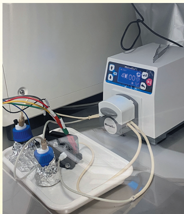
レドックスフロー電池の充放電試験
