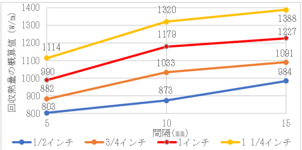
図 5 熱交換器伝熱管単位延長あたりの回収熱量 (冬季)
