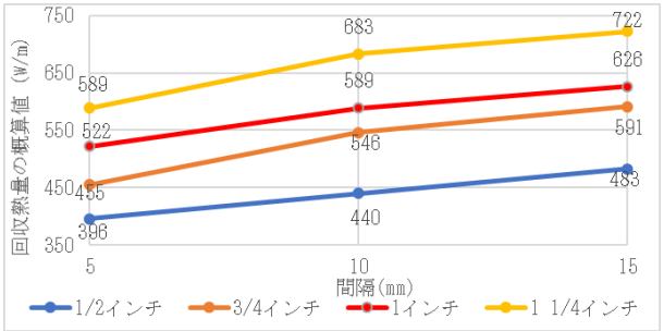
図 4 熱交換器伝熱管単位延長あたりの回収熱量 (夏季)
